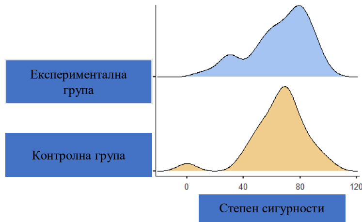
Слика 1: Функција густине степена сигурности на одабир позиције на линији за препознавање, за контролну и експерименталну групу (минимална вредност – 0; максимална вредност 100).
